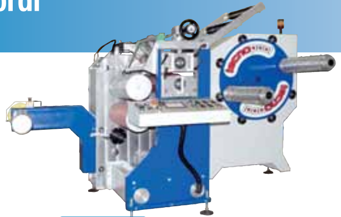
TG500 REV 500 - 750 Taglierina ribobinatrice per bordi forti spessori con due avvolgitori a revolver
